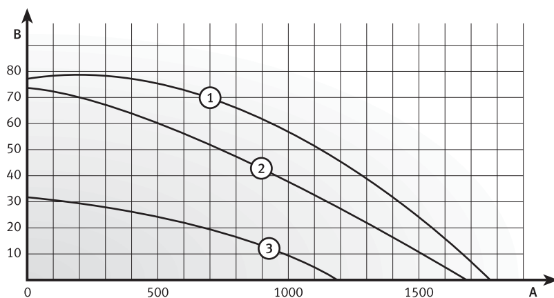
Curvas de presión disponible de la bomba del circuito de calefacción
